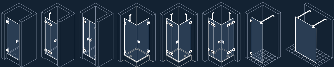
Krídlové dvere SOLVA PRO s pevným segmentom do niky šírka 700~1500 mm výška 1200~2200 mm, hĺbka no limit od 2 362,80 €
